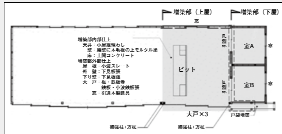
痕跡図(ピットを含む右側空間が戦時中の増改修範囲)
