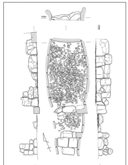
横穴式石室実測図
