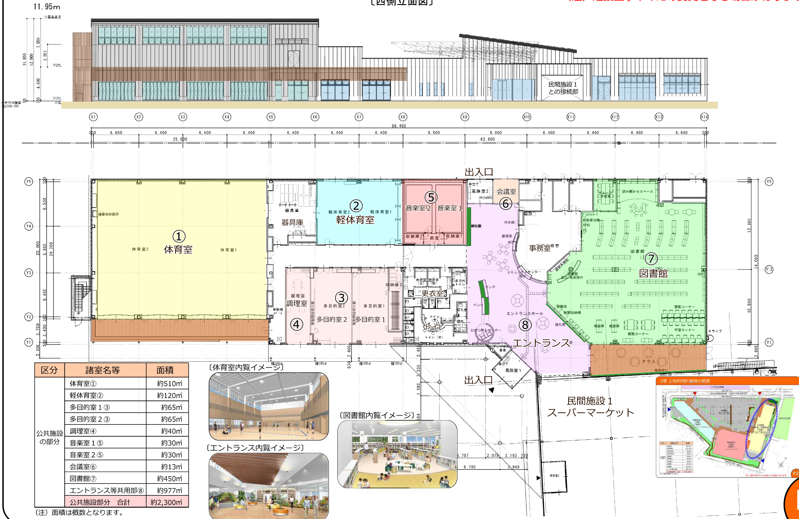
〔西側立面図〕
