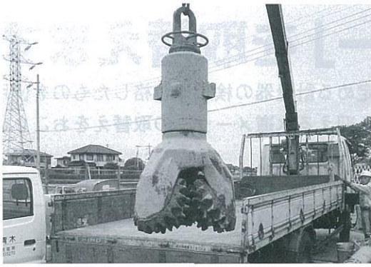
井戸の掘削ドリル先端部分
