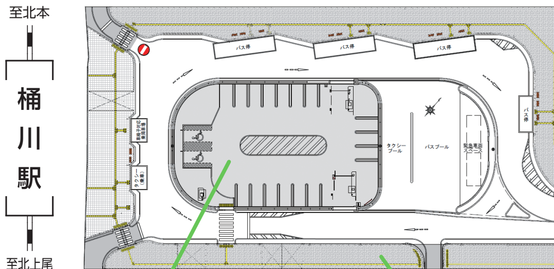
〈駅東口駅前広場平面図〉
