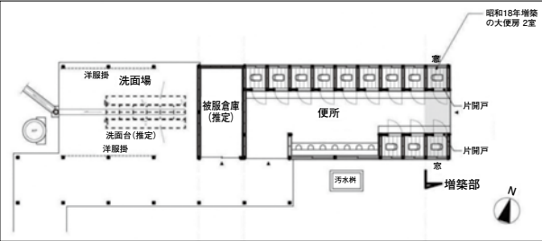
昭和18年当時の便所棟復原平面図
